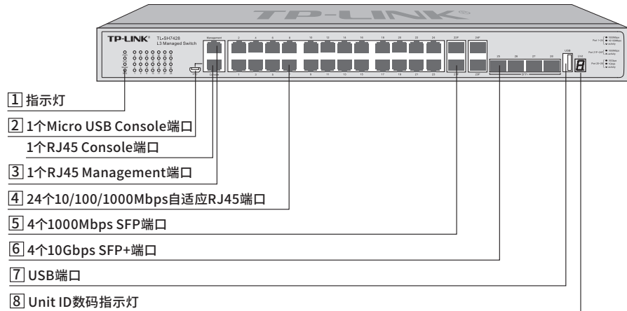
图1-4 TL-SH7428前面板示意图
