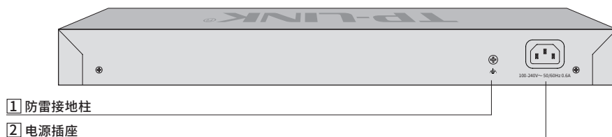
图1-8 TL-SH6428后面板示意图
