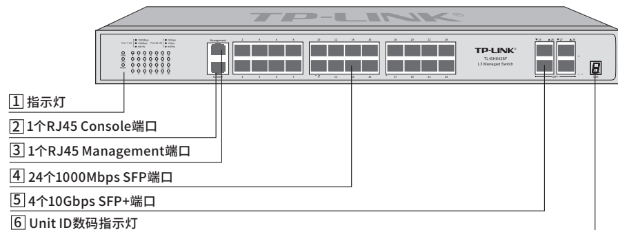
图1-3 TL-SH6428F前面板示意图
