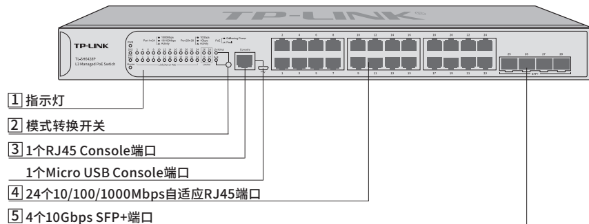
图1-2 TL-SH6428P前面板示意图
