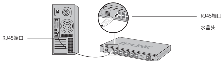
图3-1 RJ45端口连接示意图
