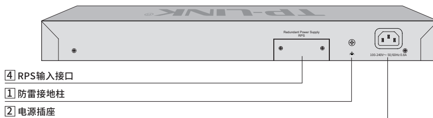
图1-11 TL-SH7428后面板示意图
