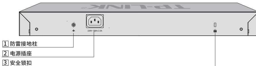
图1-10 TL-SH6428P后面板示意图
