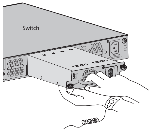
图3-7 安装电源模块示意图
