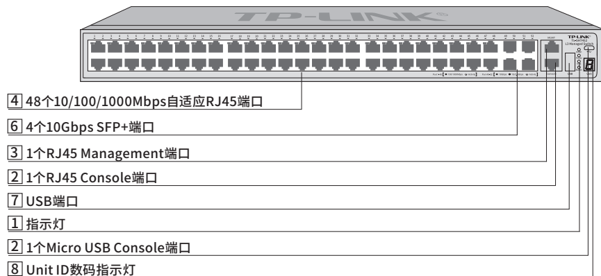
图1-6 TL-SH7452前面板示意图
