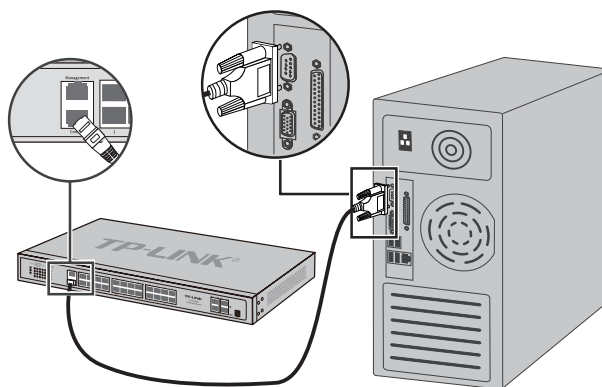
图3-3 RJ45 Console端口连接示意图
