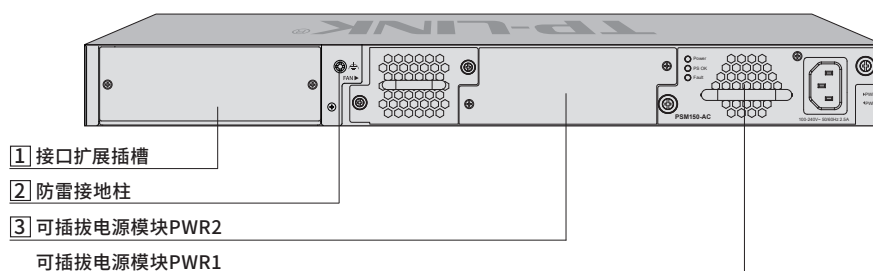
图1-13 TL-SH7452后面板示意图
