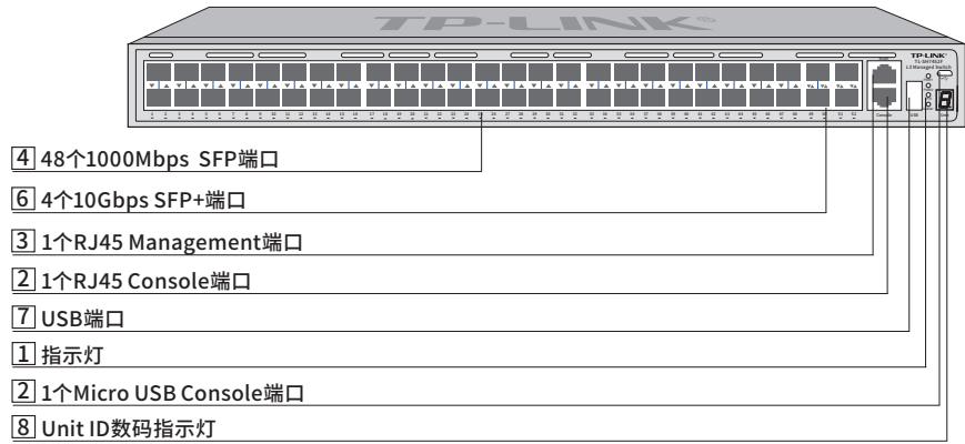
图1-7 TL-SH7452F前面板示意图
