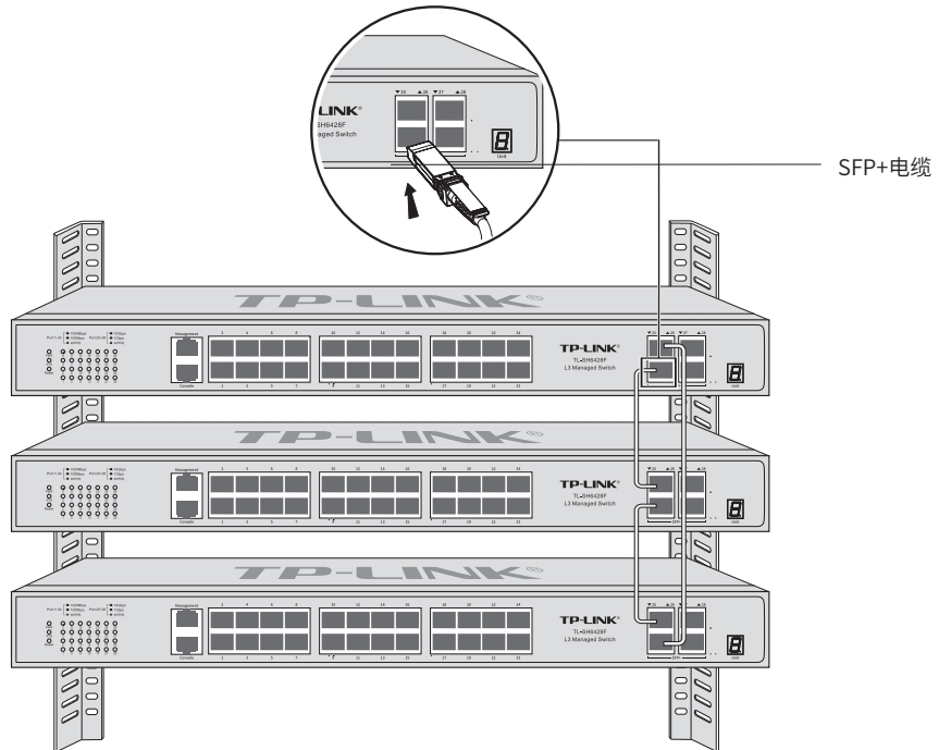
图2-4 使用SFP+端口建立堆叠示意图
