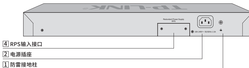
图1-12 TL-SH7428F后面板示意图
