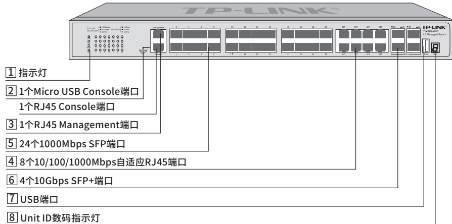
图1-5 TL-SH7428F前面板示意图
